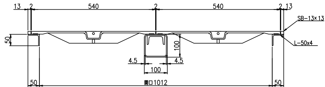
C-C断面図
