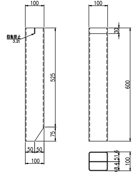
B部詳細図
