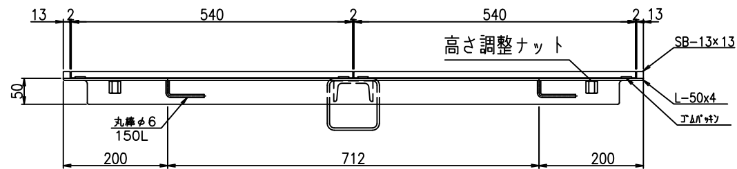
D-D断面図
