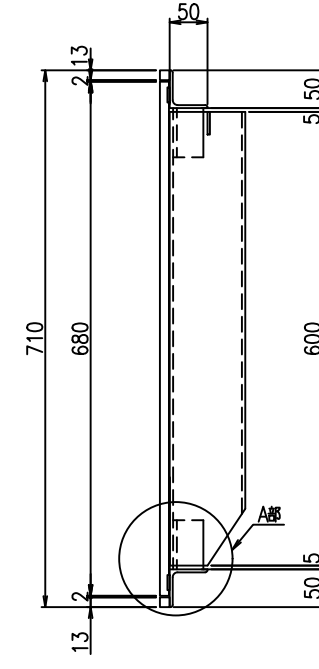
B-B断面図
